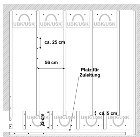
Bild 1. Anordnung von Lagerhölzern
