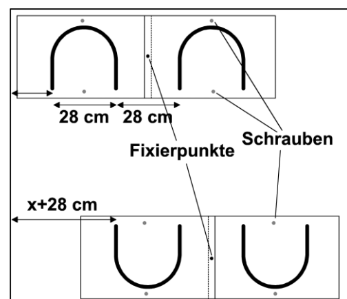
Bild 3. Befestigung der Umlenkbögen
