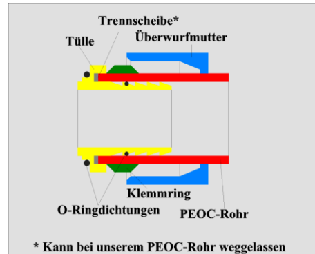
Bild 5. Heizrohr-Adapter
